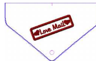
Datei: Briefumschlagklappe Vorlag....eof Stiche: 4130 Farben: 5/7 Größe: 170.1x105.0 mm Stops: 6
