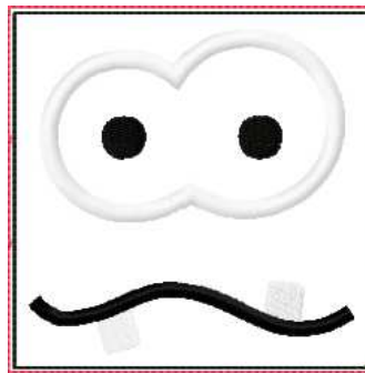
Datei: HUELLE MONSTER.vp3 Stiche: 5294 Farben: 8/15 Größe: 98.0x98.0 mm Stops: 14
